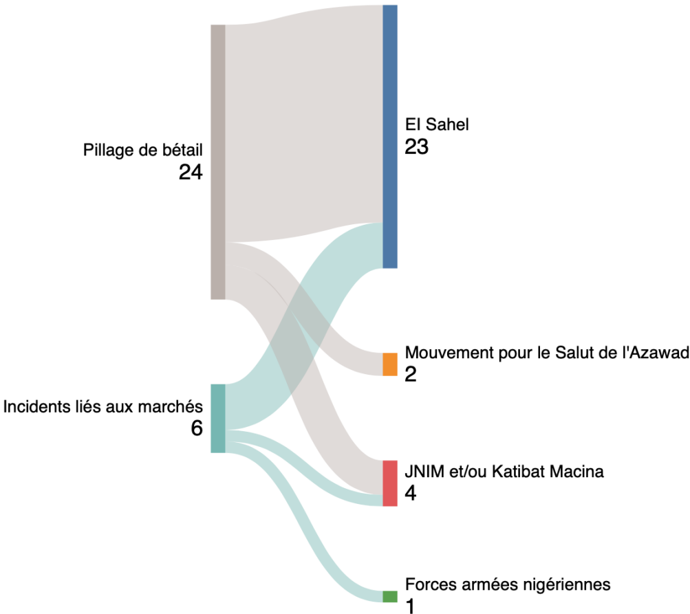
Figure 2 : Diagrammes de Sankey montrant les parties au conflit auxquelles les incidents de violence alimentaire dans la région de Ménaka ont été attribués (1er janvier 2023-30 septembre 2024).
