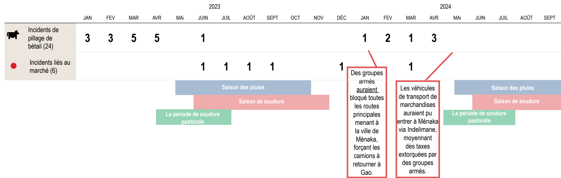
Figure 1 : Chronologie du calendrier agricole du Mali et des incidents signalés de violence liée à l’alimentation
